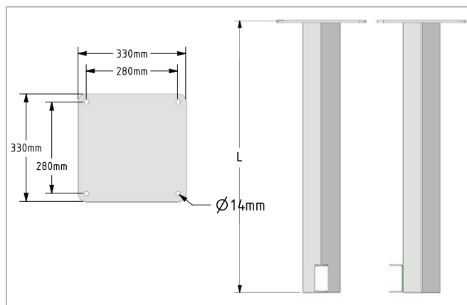
Konsol gulv/loft L=400-2500 mm. Kun til brug af ESA arm op til 5 meter.
